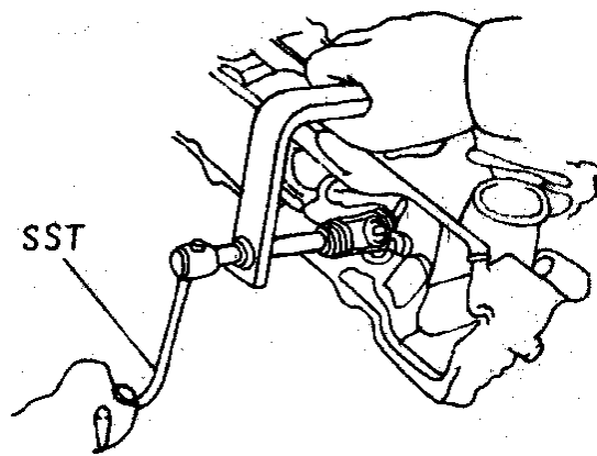
Hình3.12: Dùng cảo nén lò xo xupap
