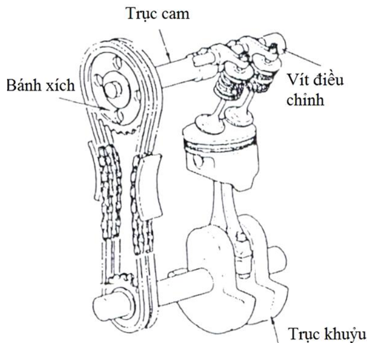
Hình 2.3: Canh khe hở nhiệt xupáp
