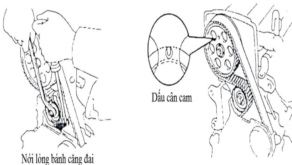
Hình 1.9: Xác định dấu trục cam
