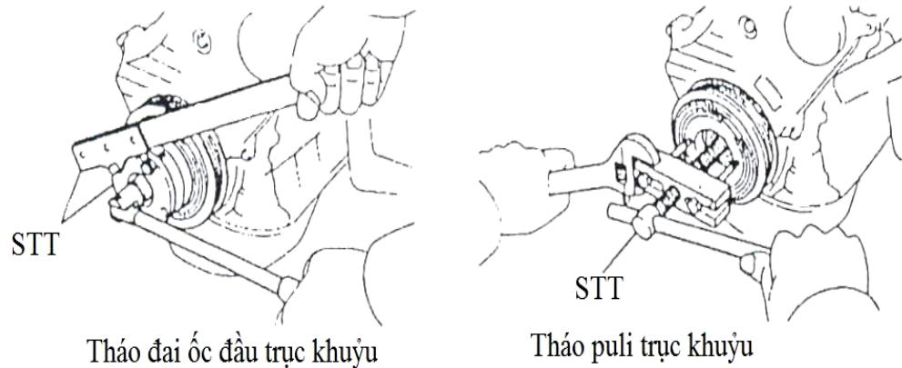
Hình 1.10: Dùng cảo tháo puli đầu trục khuỷu và tháo nắp đáy mặt dưới.
