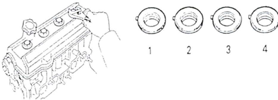
Hình 1.13: Tháo nắp đậy trực cam ở trên nắp máy.
