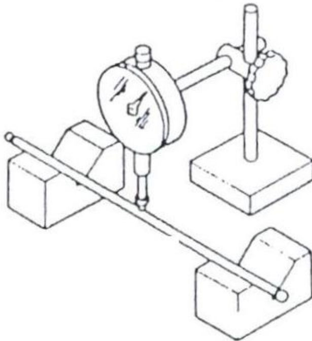
Hình 4.7: Kiểm tra đĩa đẩy
